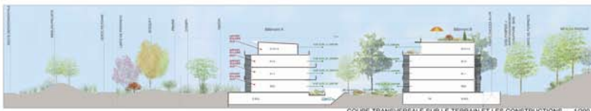
COUPE TRANSVERSALE SUR LE TERRAIN ET LES CONSTRUCTIONS - 1/200
